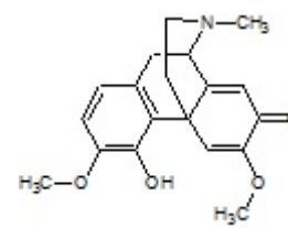
Salutaridine
