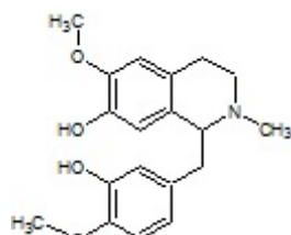
Reticuline
